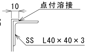
C部詳細図
