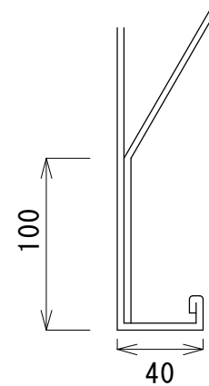
A部詳細図
